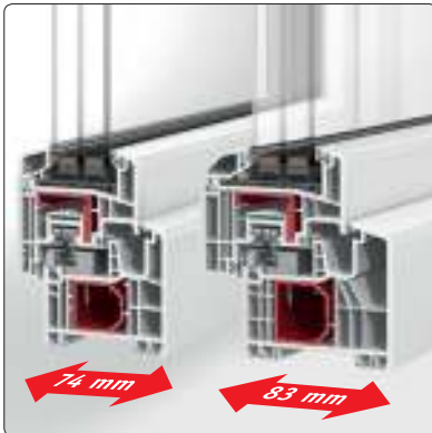
Vergleich Bautiefe PaXabsolut 74/83mm
