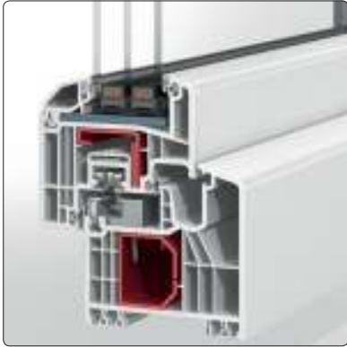
PaXabsolut83 flächenversetzt, auch in 74 Millimeter Bautiefe erhältlich
