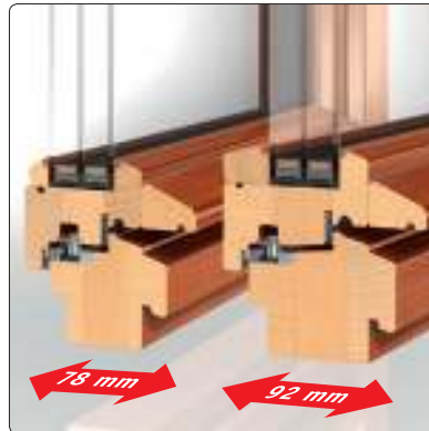
Vergleich Bautiefe PaXcontur 78/92 mm
