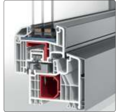
PaXabsolut83 Alublend flächenversetzt, auch in 74 Millimeter Bautiefe erhältlich
