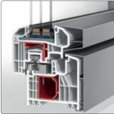
PaXabsolut83 Alublend flächenbündig, auch in 74 Millimeter Bautiefe erhältlich
